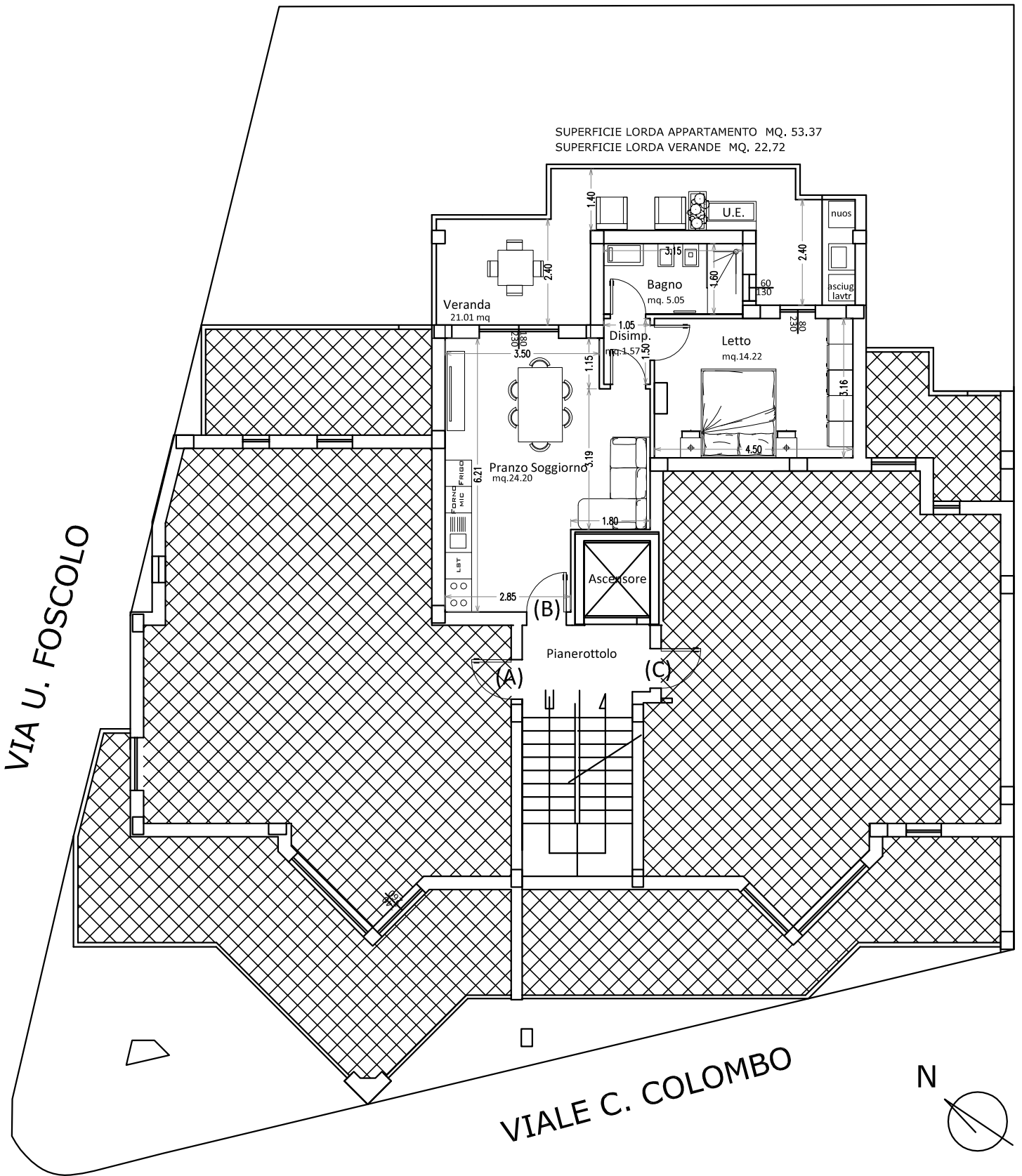
PIANO SECONDO SC. 1:100
