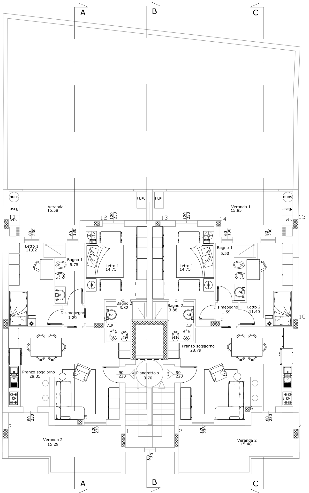
Pianta Piano secondo e terzo arredata sc. 1:100
